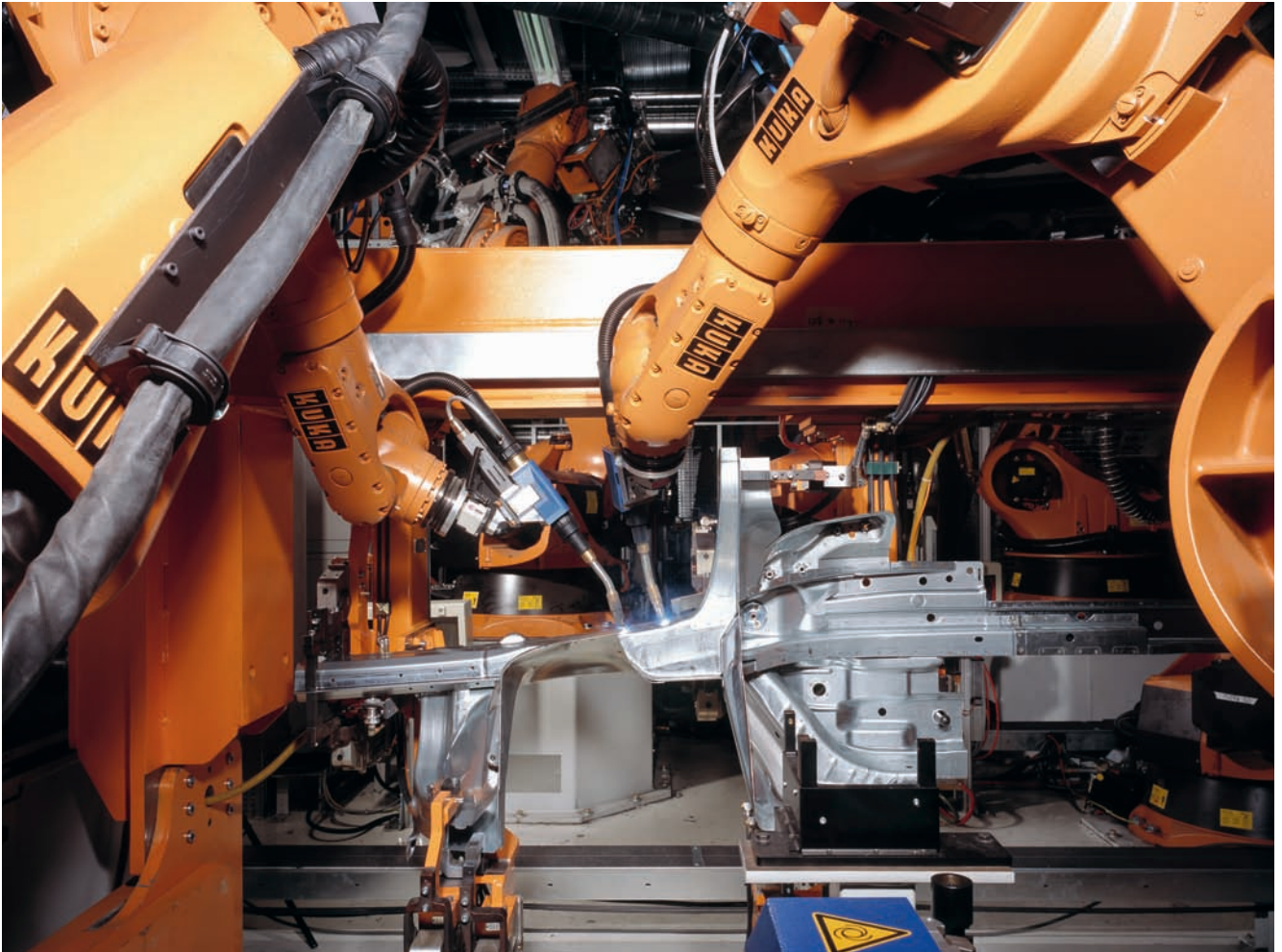
Audi AG – Schweißroboter
